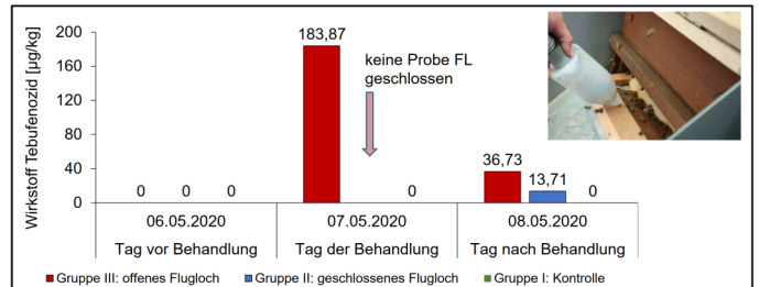
Abb. 5: Rückstände in heimkehrenden Sammlerinnen am Tag vor der Behandlung, am Behandlungstag und am Tag nach der Behandlung.
